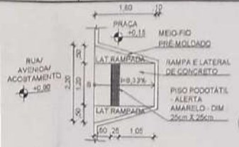
5 PL. BAIXA - DET. TÍP. DAS RAMPAS ESCALA: 1:50
