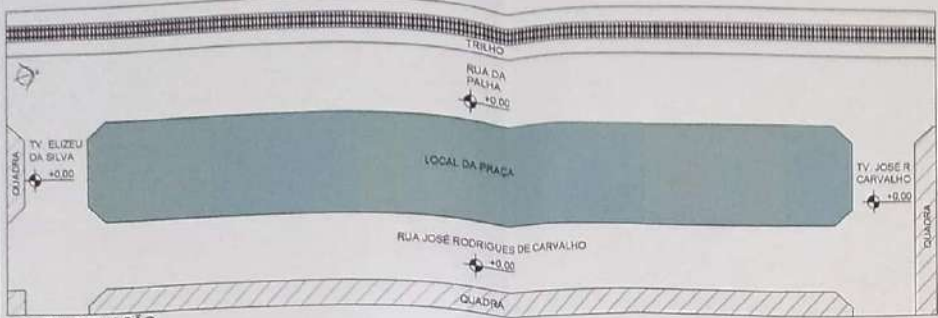
1 PL. SITUAÇÃO ESCALA: 1:300
