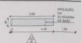
6 PL. BAIXA - DET. TÍP. DOS BANCOS ESCALA: 1:50
